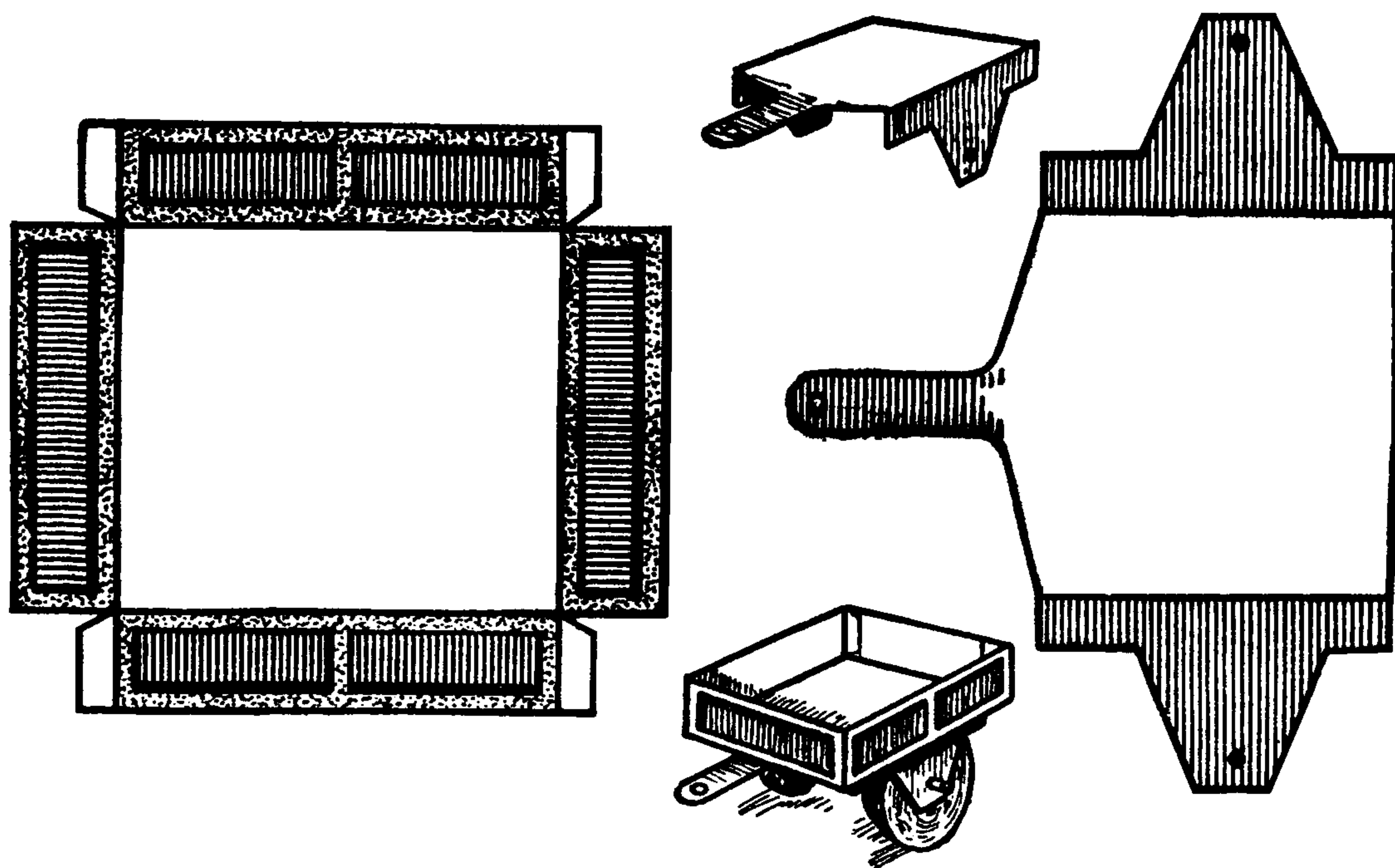
Кузов и рама модели двухколёсного прицепа.
