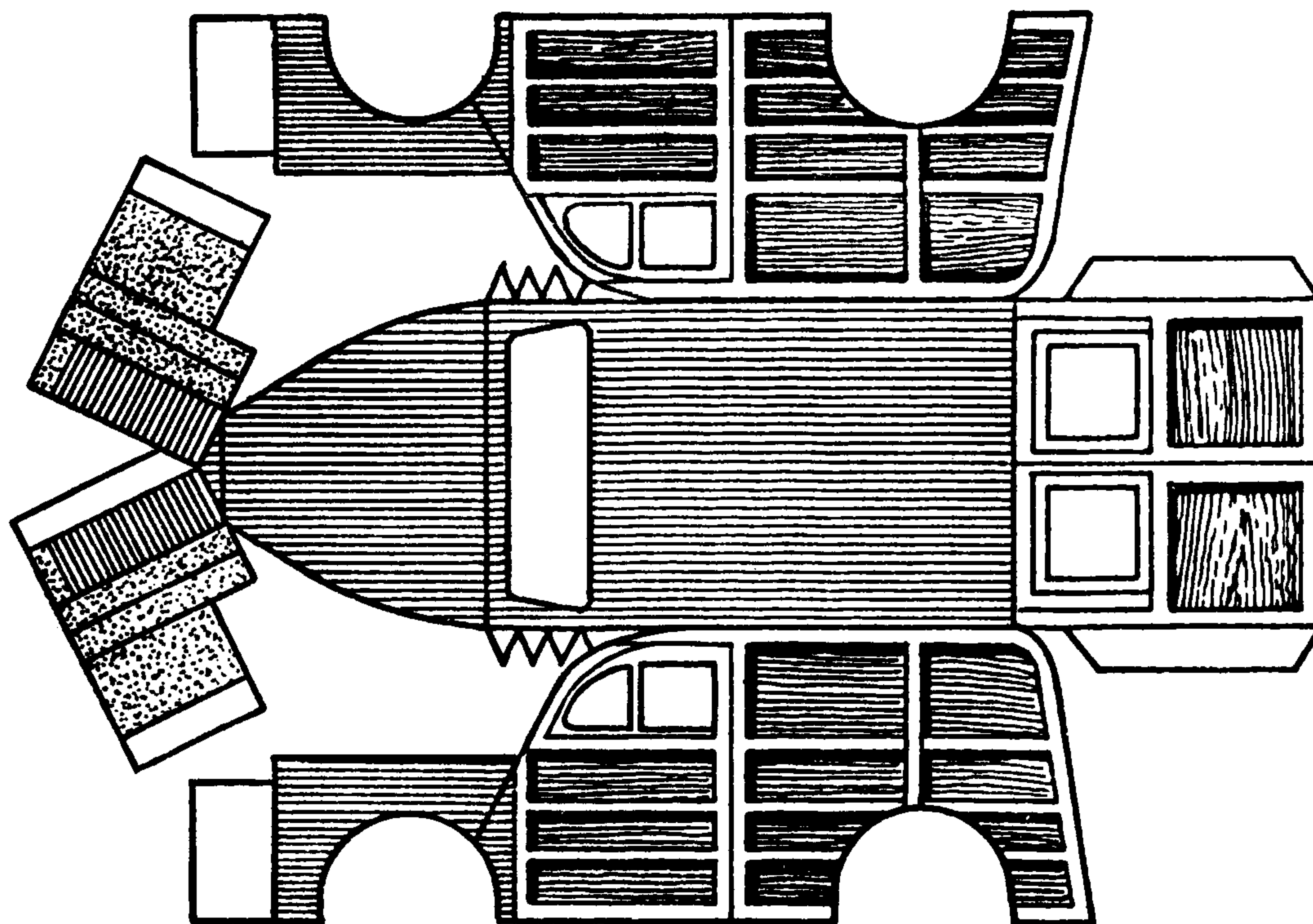
Кузов модели «Москвич»-фургон.
