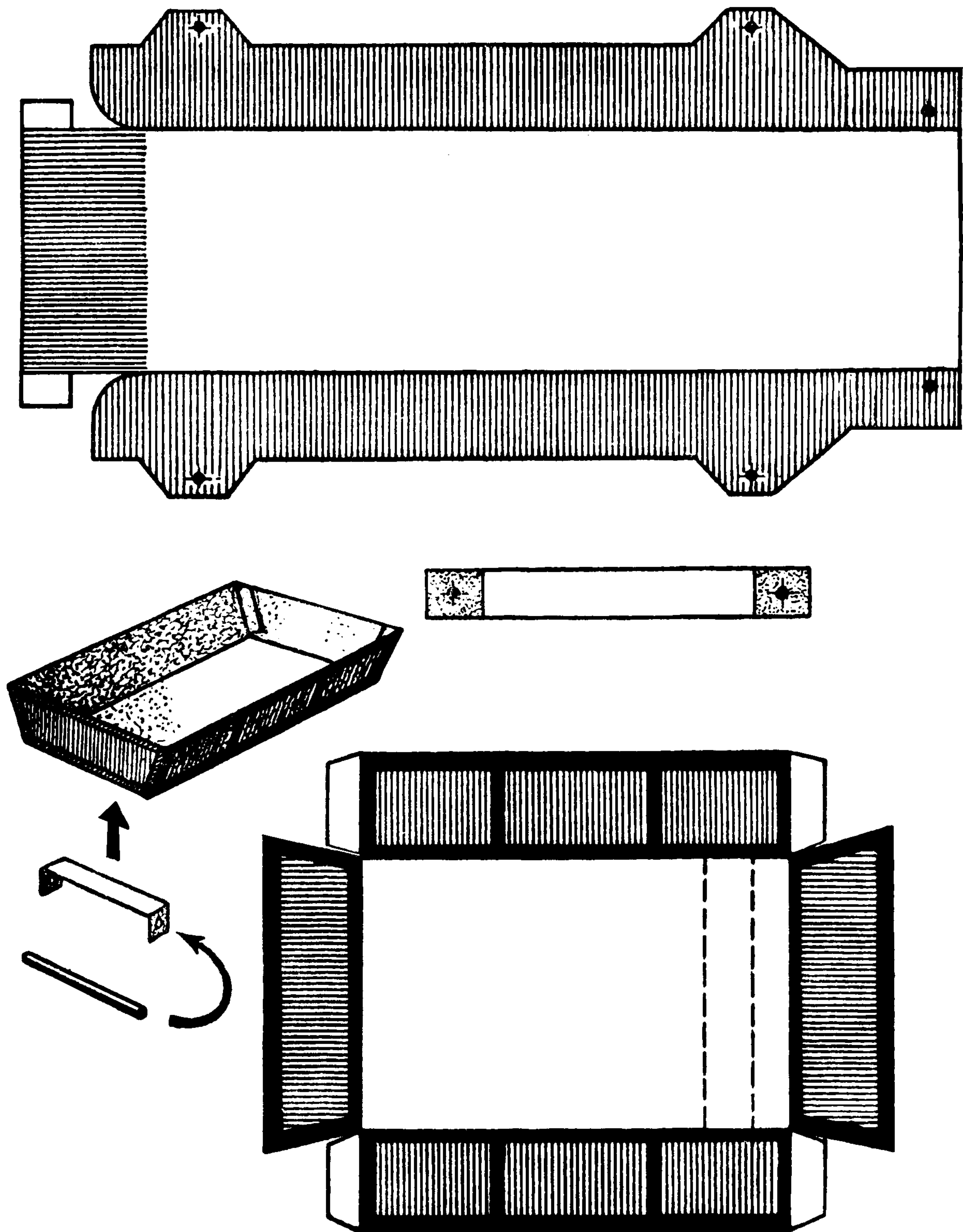
Рама самосвала, кузов и скобка.
