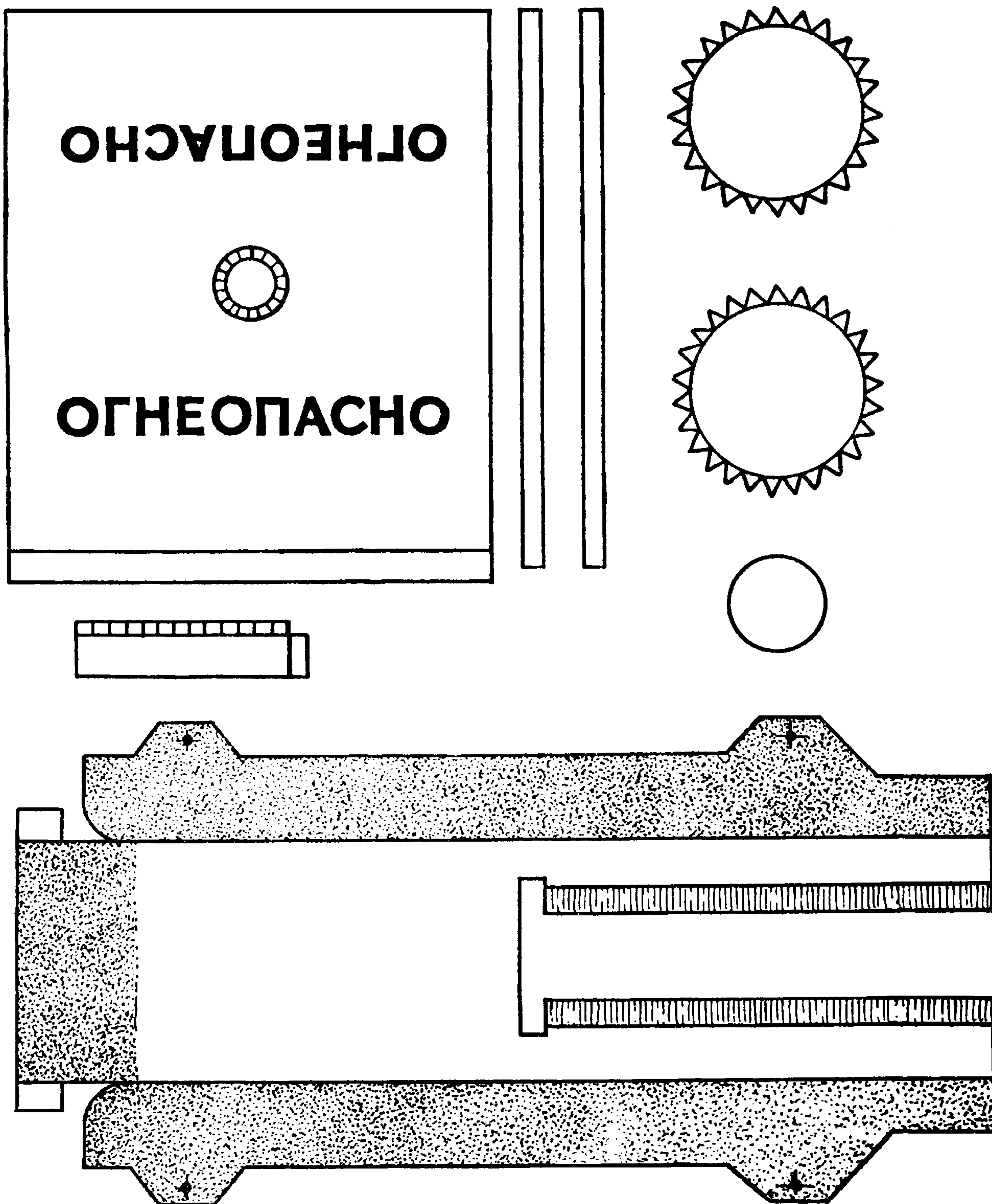
Рама автоцистерны, горловина, труба и донья.
