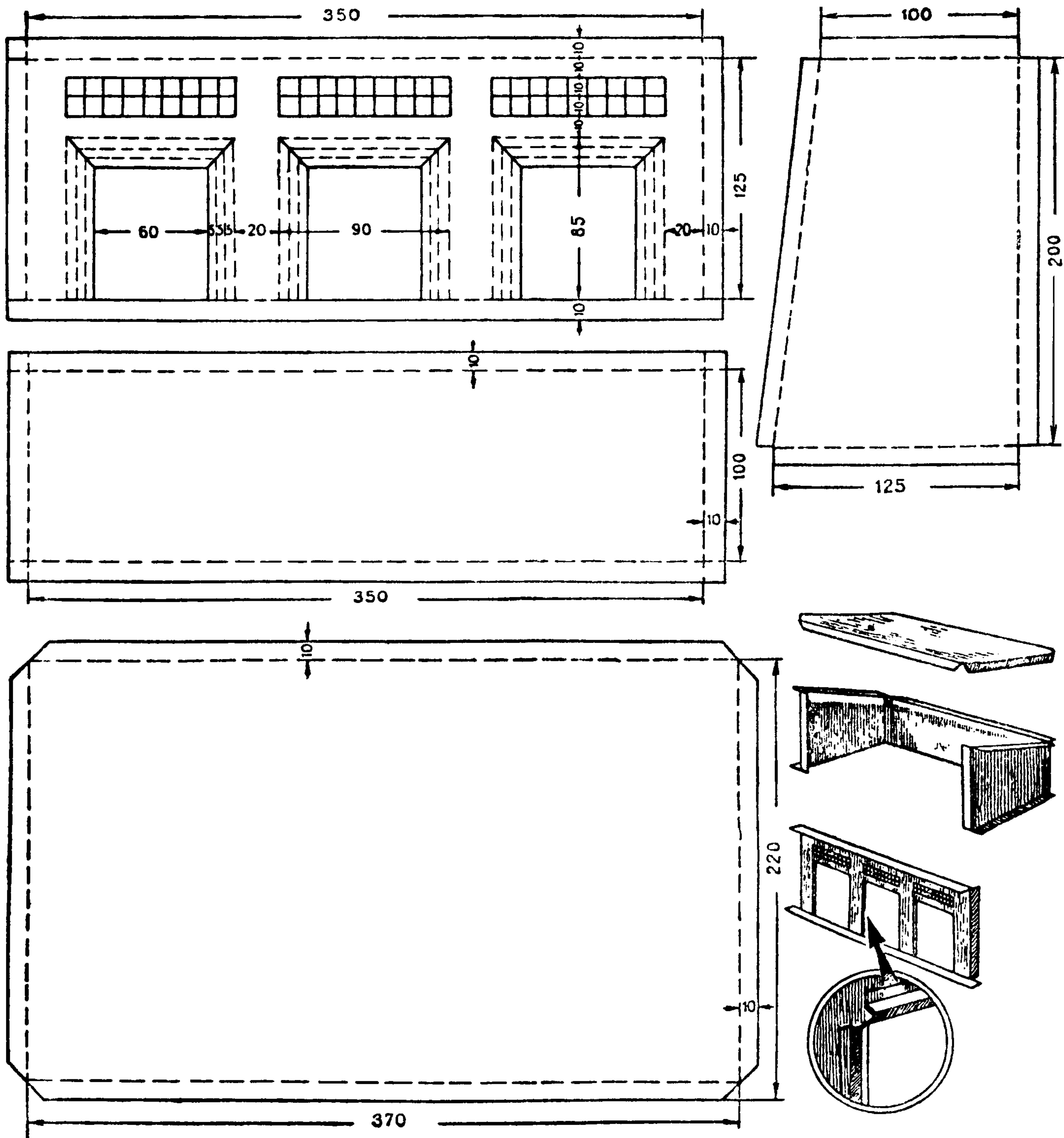
Стенки и крыша модели гаража.
