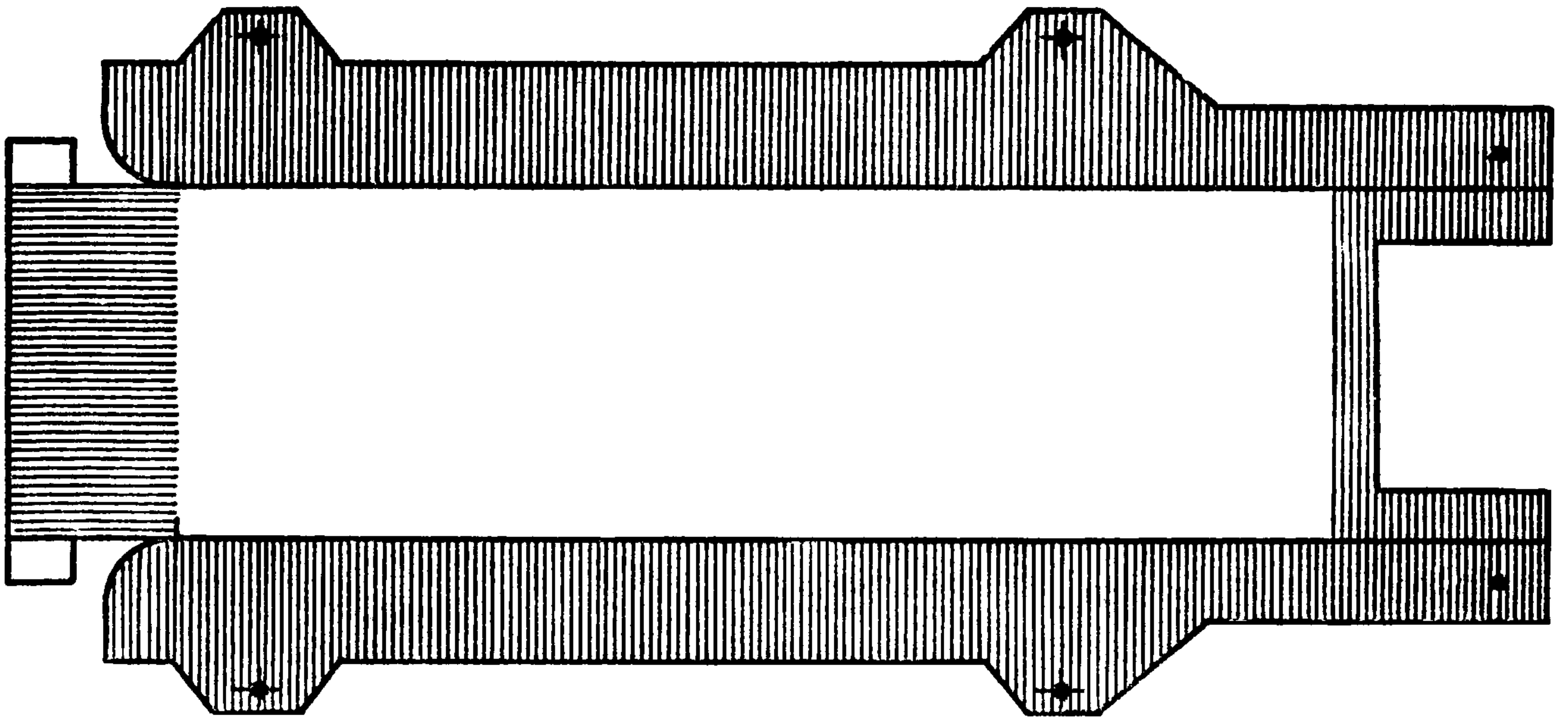
Рама модели пожарной машины.
